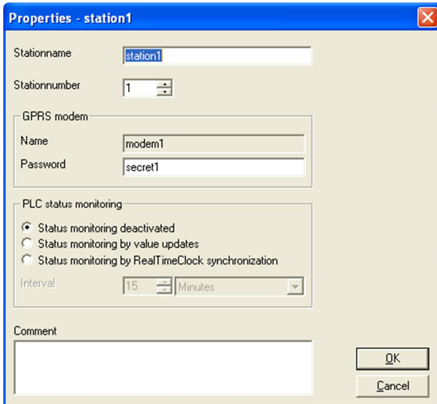
图 22 站的配置
