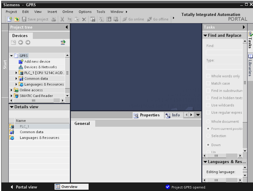
图 28 项目视图
